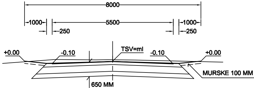
POIKKILEIKKAUKSET 1:100 PLV 0 ... 250
