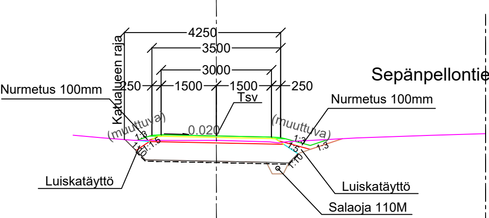
POIKKILEIKKAUS 1:100 PLV. 532-587 JA 672-852
