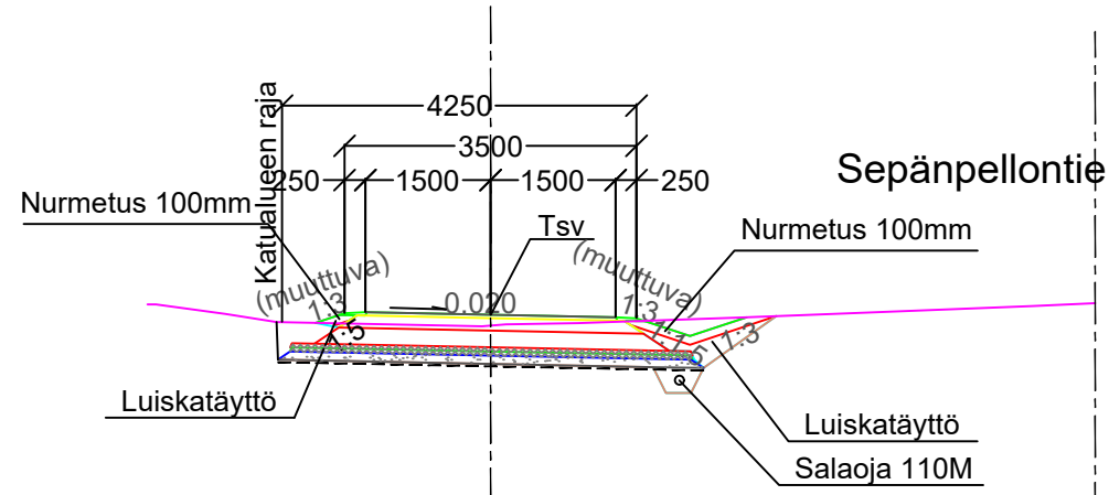
POIKKILEIKKAUS 1:100 PLV. 587-672
