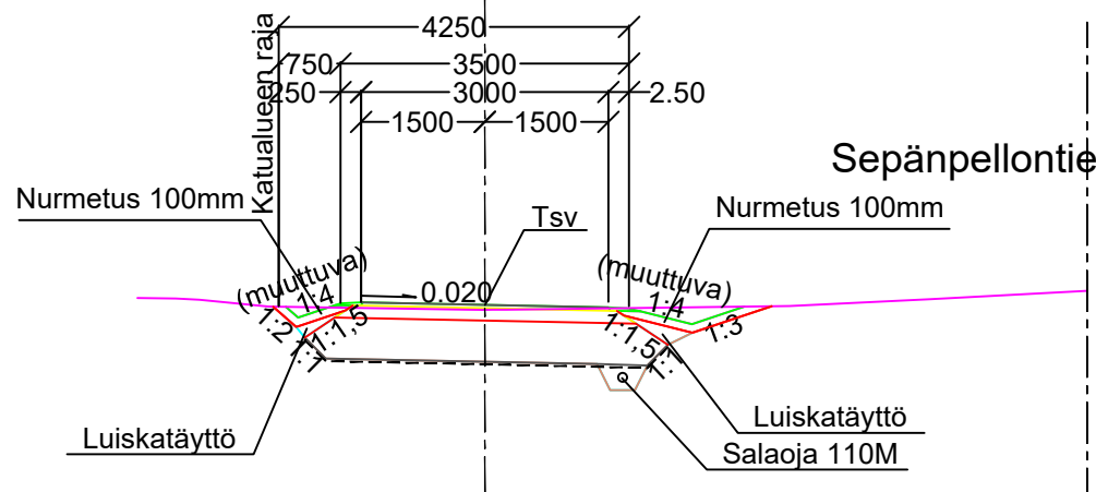
POIKKILEIKKAUS 1:100 PLV. 477-532 ja 852-892.34
