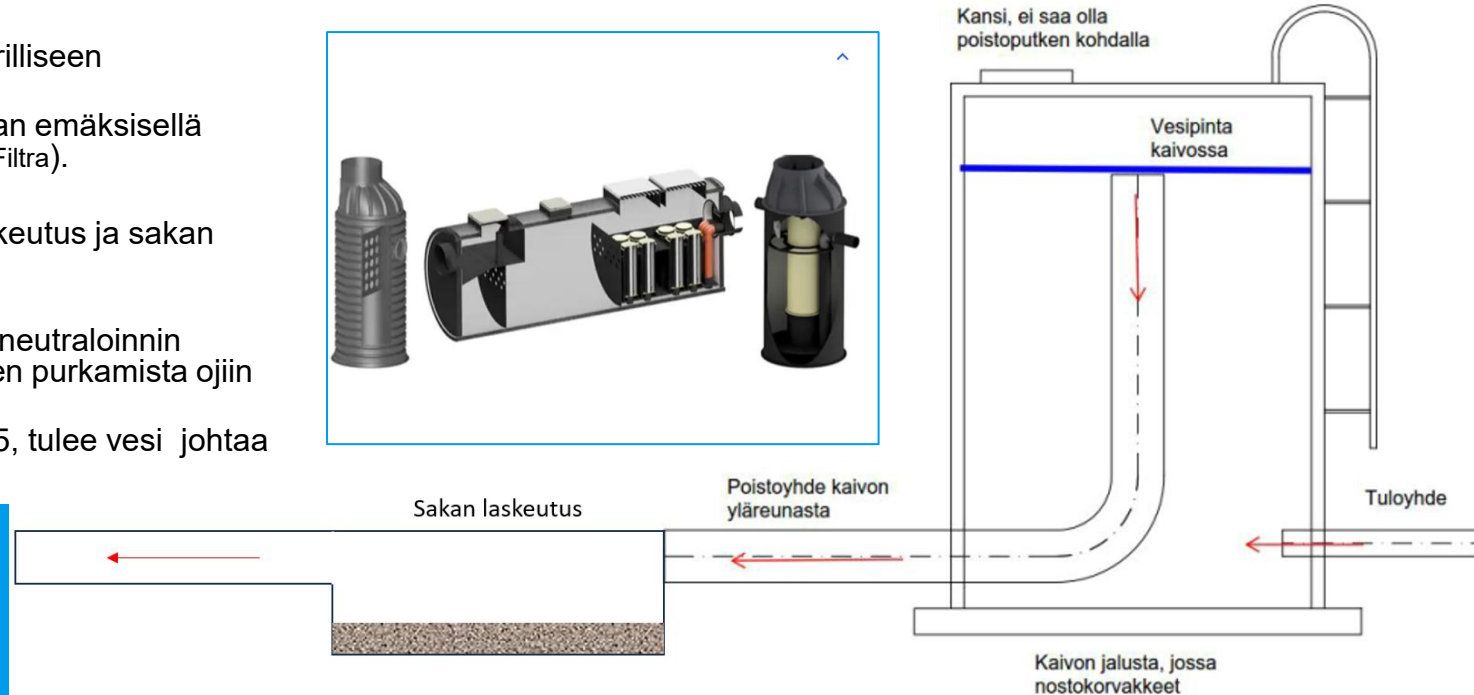
Kuva 4: Tyypikuva neutralointikaivosta.
